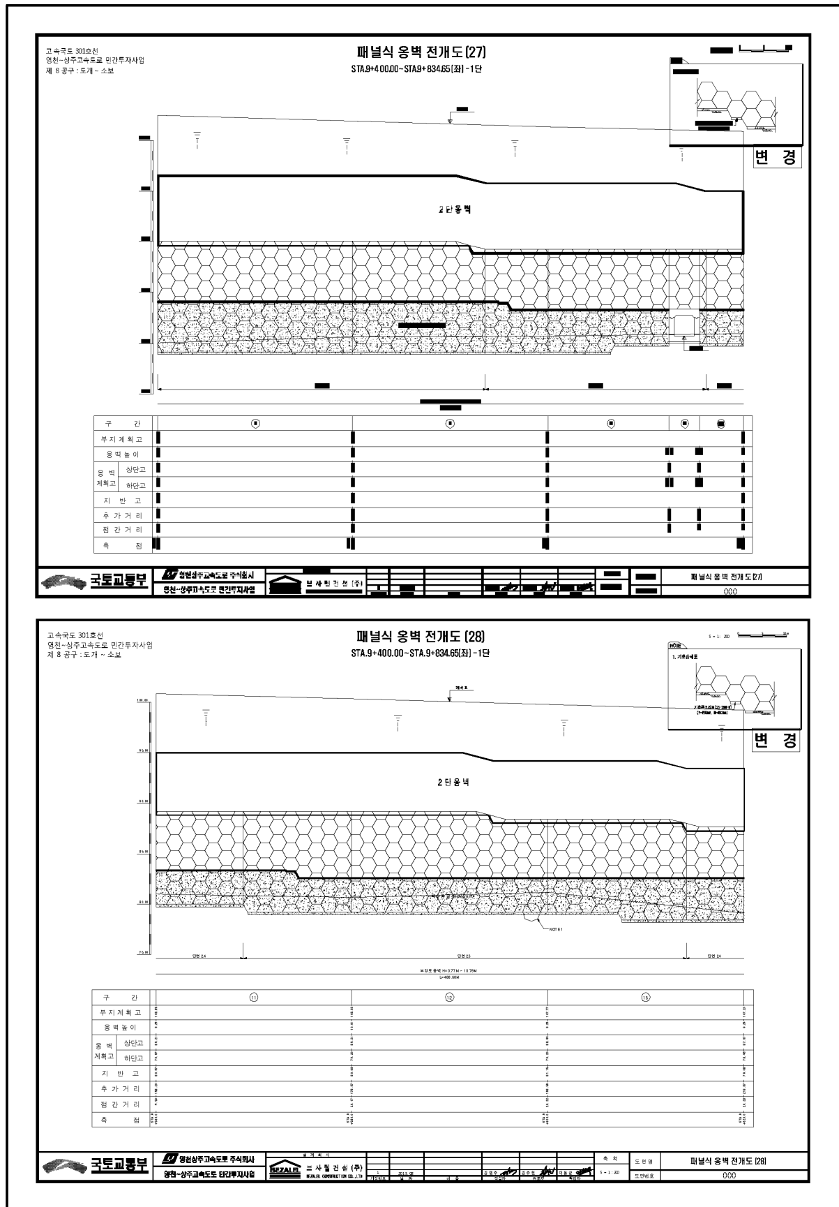
【그림 2.4】 전개도(계속)
