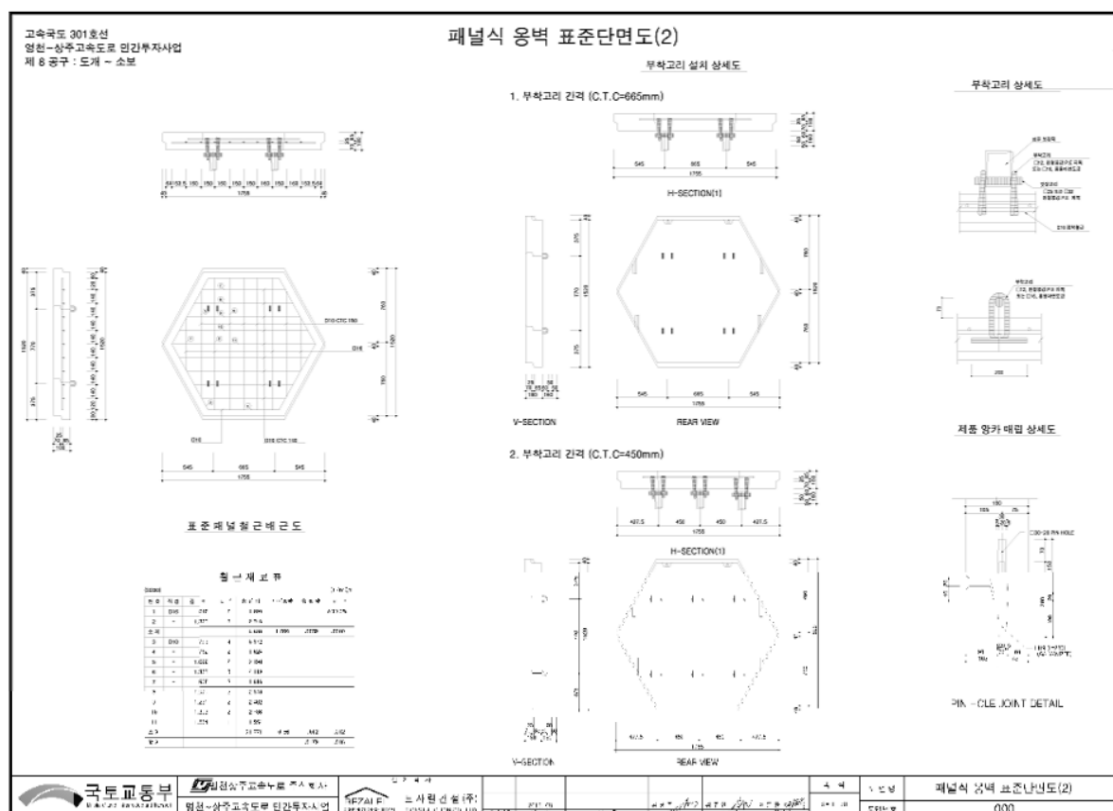
【그림 68.5】 단면도
