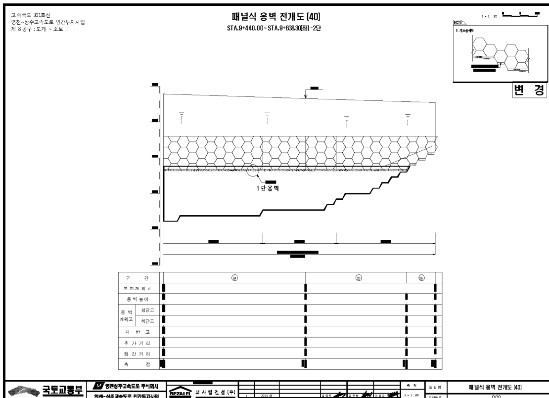
【그림 2.4】전개도(계속)
