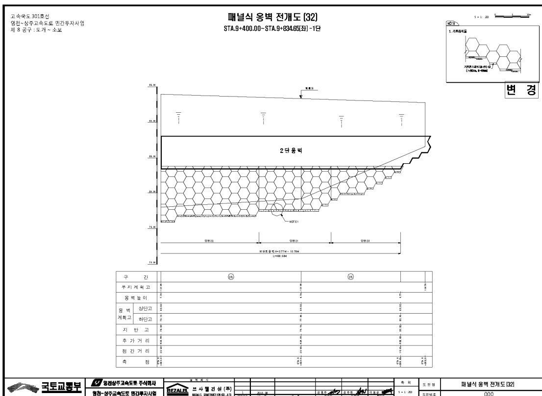
【그림 2.4】전개도(계속)
