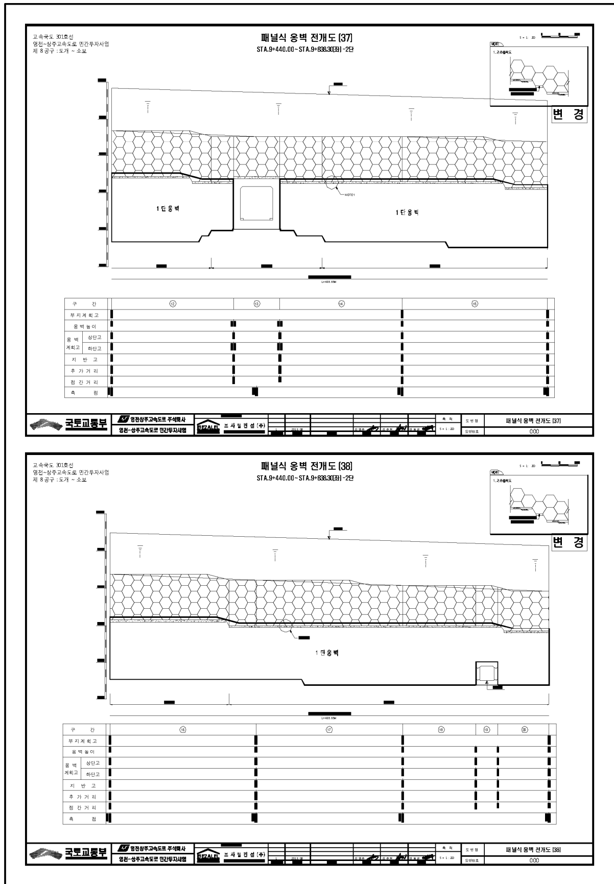
【그림 2.4】 전개도(계속)
