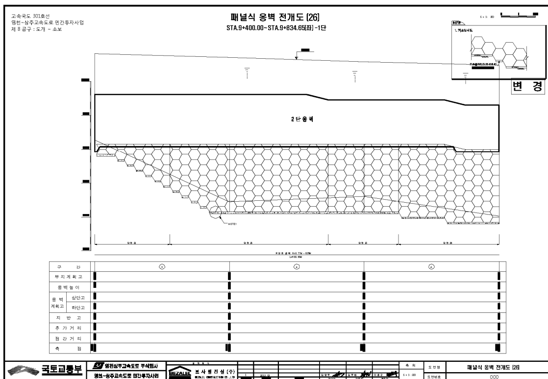
【그림 68.4】전개도
