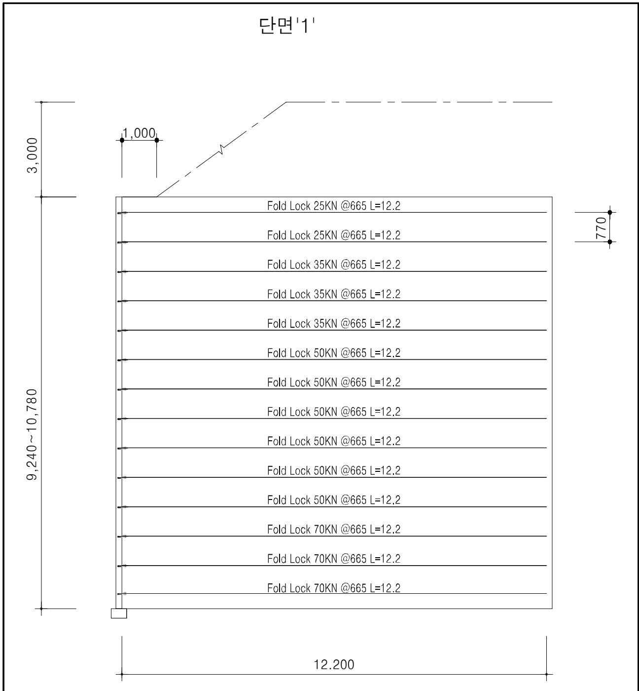
【그림 68.10】 검토단면도
